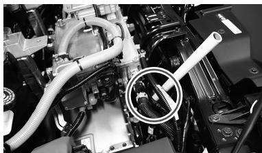
フロント電動機型式位置 (棒先・AM67)
